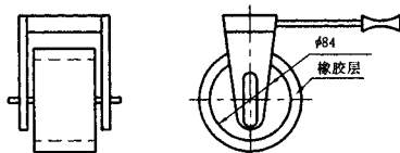
图 1 压辊示意图
